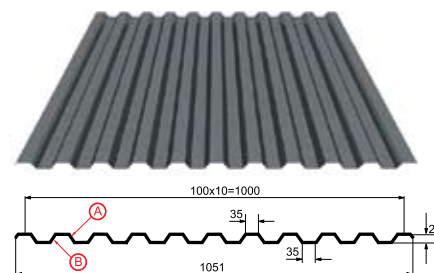
Профилированный лист С-21x1000-А
