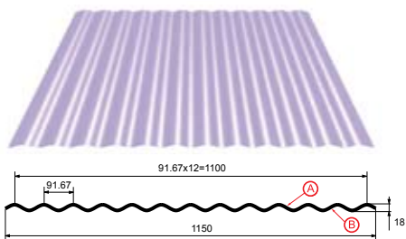
Профилированный лист МП-18x1100-А "Волна"
