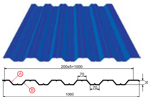
Профилированный лист НС-35x1000-А
