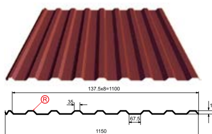
Профилированный лист МП-20x1100-Р
