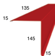
Планка торцевая 135x145x2000
