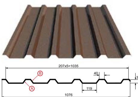
Профилированный лист МП-35x1035-В
