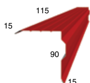
Планка торцевая 90x115x2000
