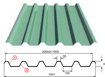
Профилированный лист С-44x1000-А
